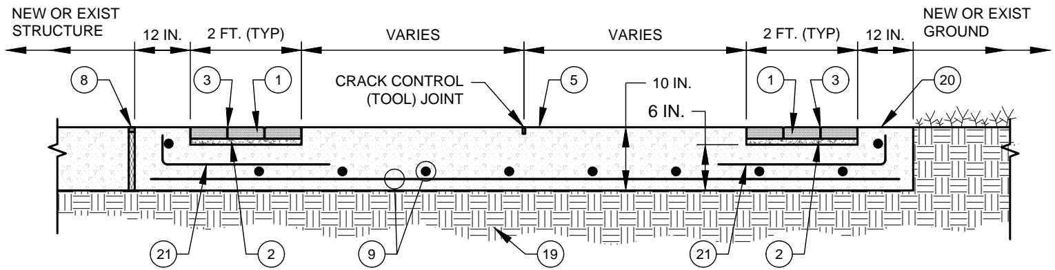
SECTION A-A
