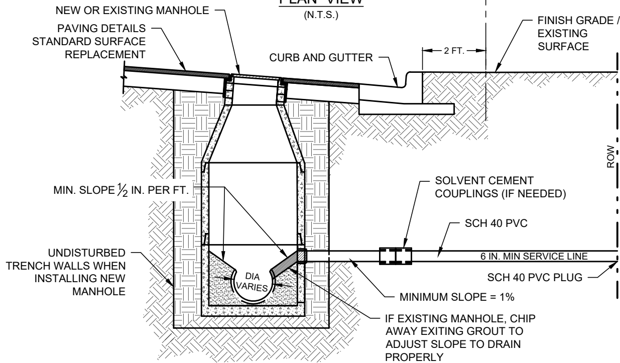
SECTION VIEW (N.T.S.)
